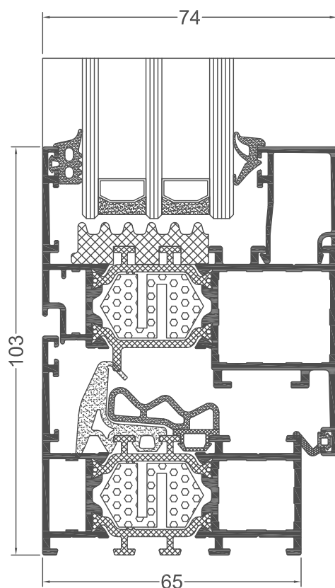
przekrój przez okno GR 65 (GR010 + GR020)
