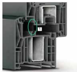
1 uszczelka środkowa
