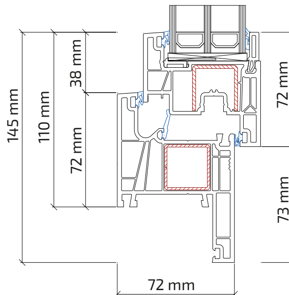
okno renowacyjne - płetwa 35 mm
