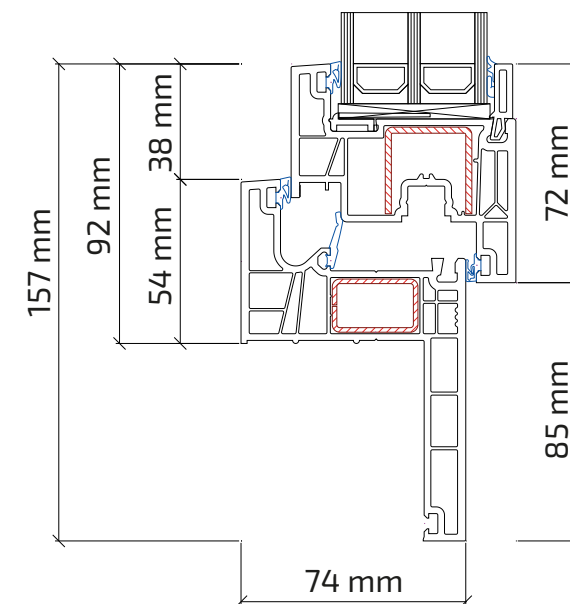
okno renowacyjne - płetwa 65 mm
